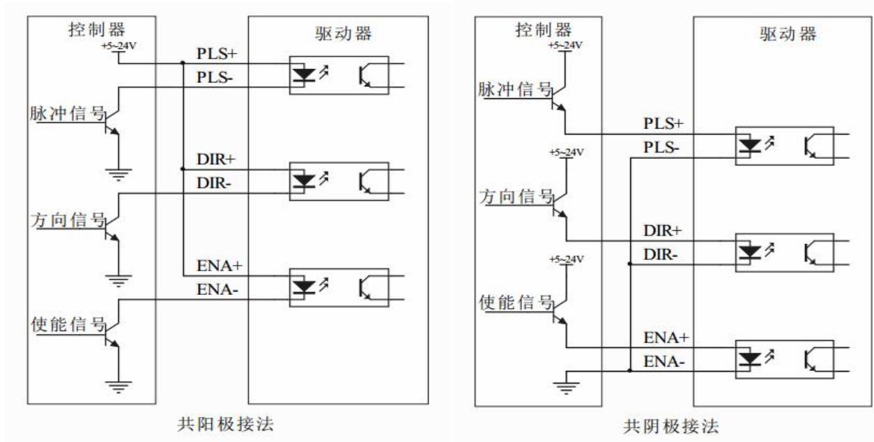
图2 输入接口电路
