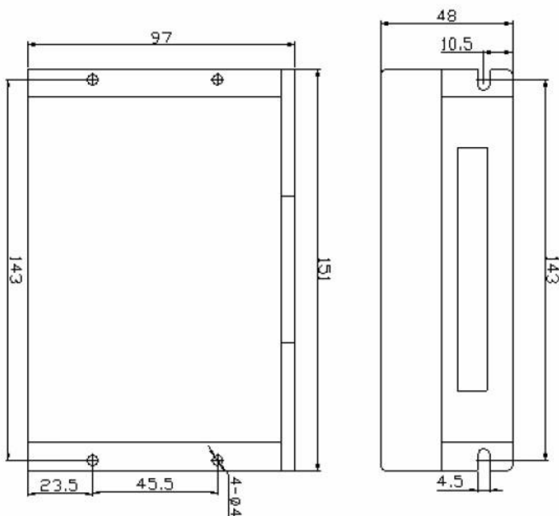
正面安装图
